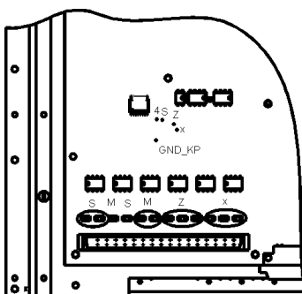
Рисунок 2.5 - Установка съемных перемычек для подключения импульсных датчиков с питанием +5В
