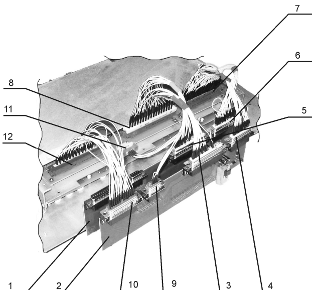
Рисунок 6.2. – Внешний вид Модуля МПУ МС-2109 с подключенными блоками самотестирования (фрагмент)
